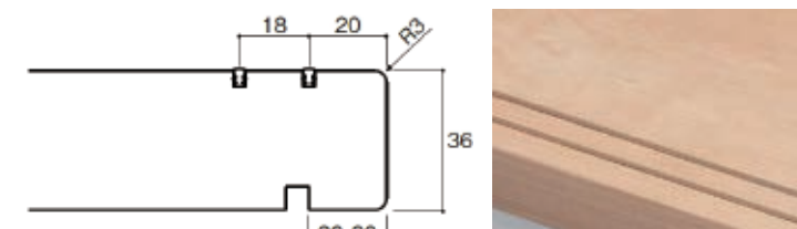
踏板断面 踏板厚：36mm 鼻の出：20mm標準
